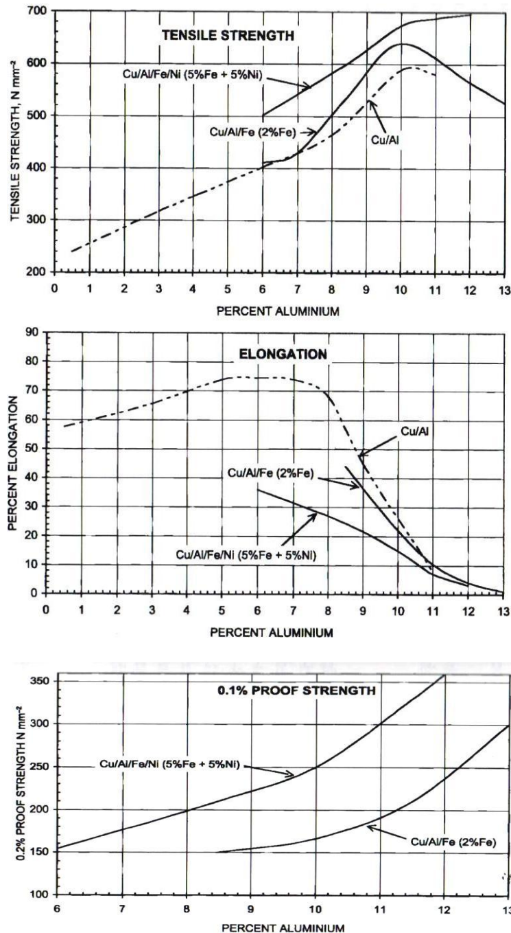
Fig. 2.2.1.1 Sammenhængen mellem mekaniske egenskaber og aluminiumsindhold i tre Aluminiumbronzelegeringer.
